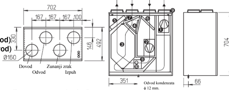
Slika: KWL EC 500 Pro R, desna izvedba naprave
