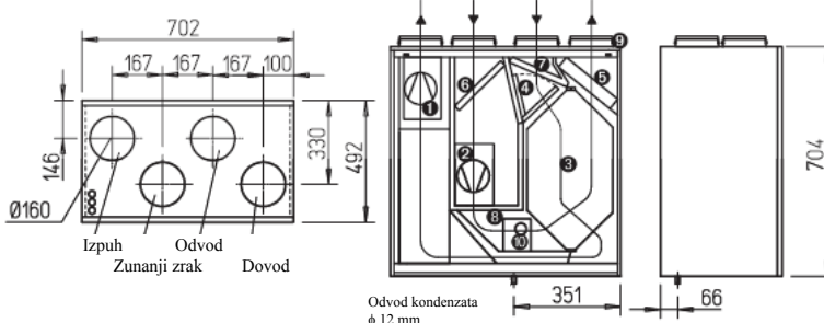
Slika: KWL EC 500 Pro L, leva izvedba naprave
